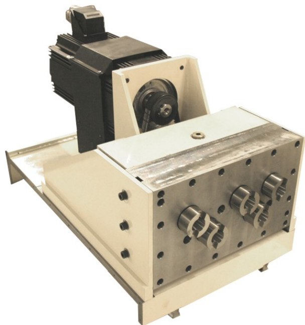
Abbildung zeigt einen 5-fach-Mehrspindelgetriebebohrkopf Sk30.
