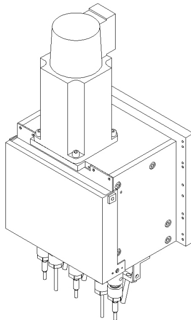
Abbildung zeigt einen 5-fach Mehrspindelbohrkopf. Der Servomotor kann als Option bestellt werden.
