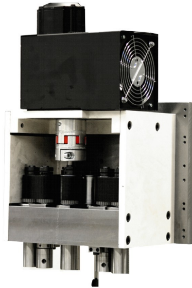
Abbildung zeigt einen 5-fach Mehrspindelbohrkopf. Der Servomotor kann als Option bestellt werden.
