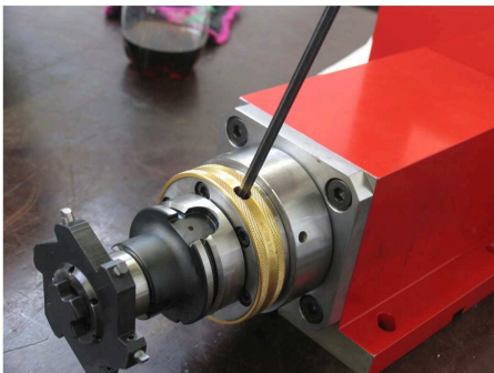
Frässpindel mit HSK 63 Werkzeugaufnahme
