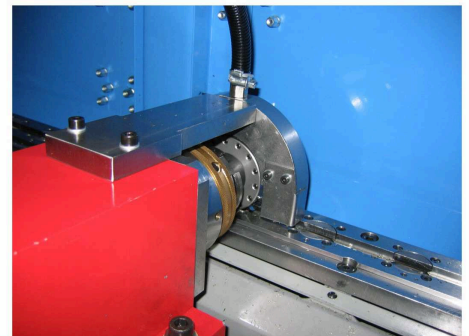
Werkzeugschmierung mit Minimalmengenschmiersystem
