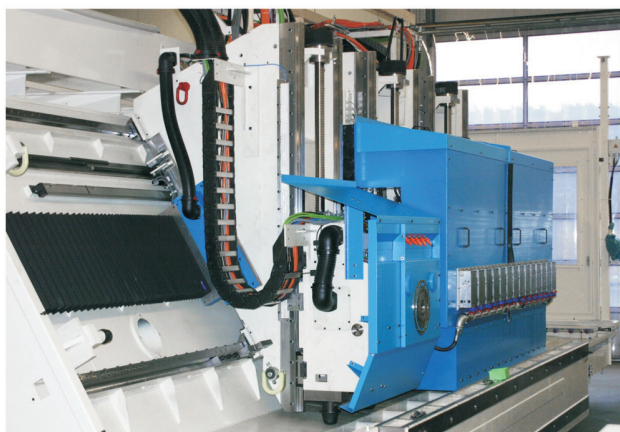
15 - Fach Präzisionsfräsmaschine mit integriertem Bearbeitungszentrum
