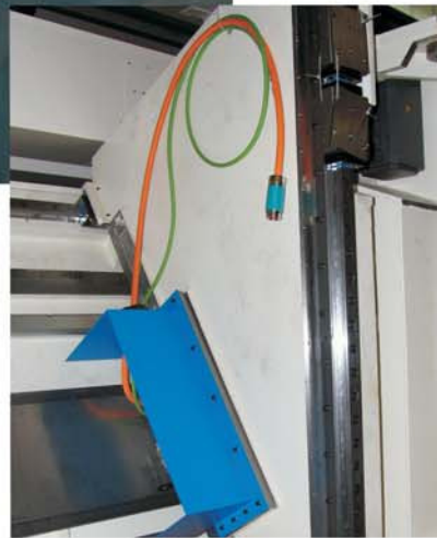
Stabile spannungsarm geglühte Schweißkonstruktion mit Beton ausgegossen
